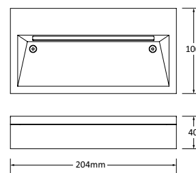
APPLIQUE - 102801.94
