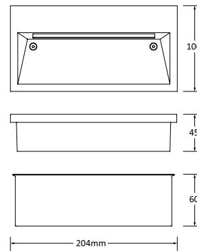
INCASSO/RECESSED - 102802.94
