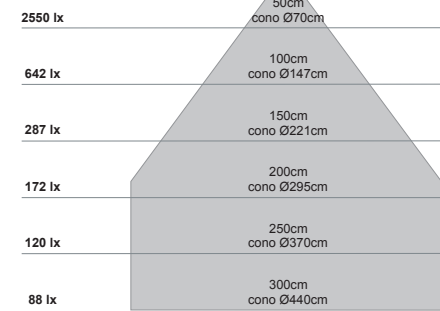
Raso Mini
